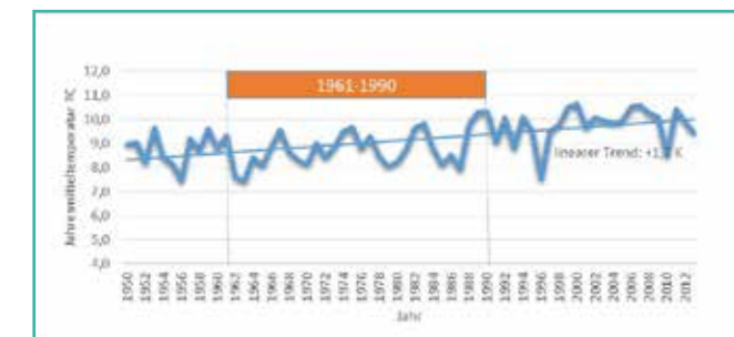
Abbildung 1: Jahresmitteltemperaturen © Hannover-Langenhagen 1950 – 2013
